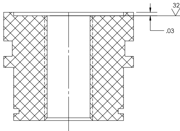
SECTION G-G SCALE 2:1
